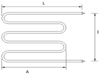
PARRILLA SALIDA LATERAL
