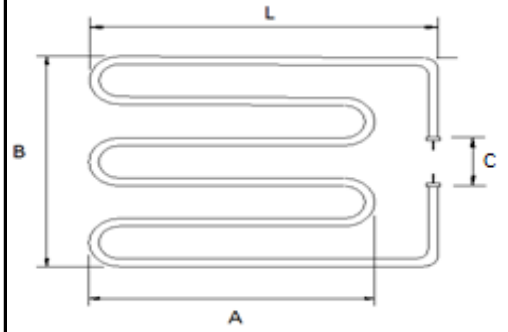
PARRILLA SALIDA HACIA ADENTRO A 90°
