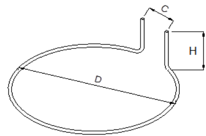
CIRC SALIDA HACIA ADENTRO A 90°
