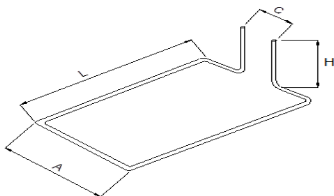
CUADRADA SALIDA HACIA ADENTRO A 90°
