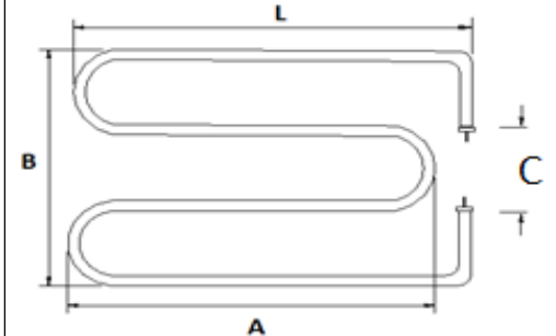
M SALIDA HACIA ADENTRO A 90°
