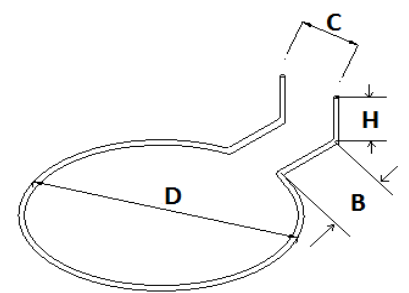
CIRCULAR SALIDA HACIA ADENTRO
